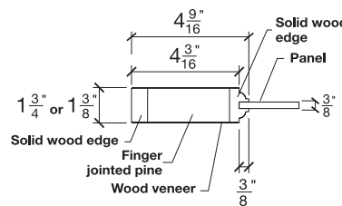
SIDERRAIL
