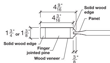
SIDERRAIL
